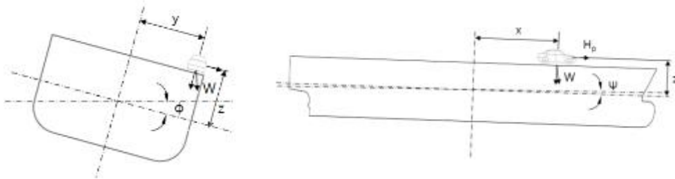
그림 1 선체운동
