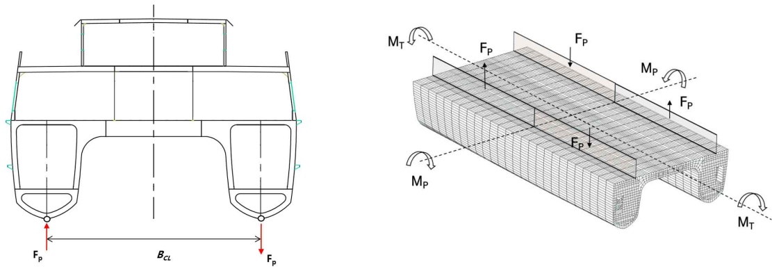
그림 3.1.5 중/횡 비틀림모멘트를 위한 중등요 연결힘 적용
